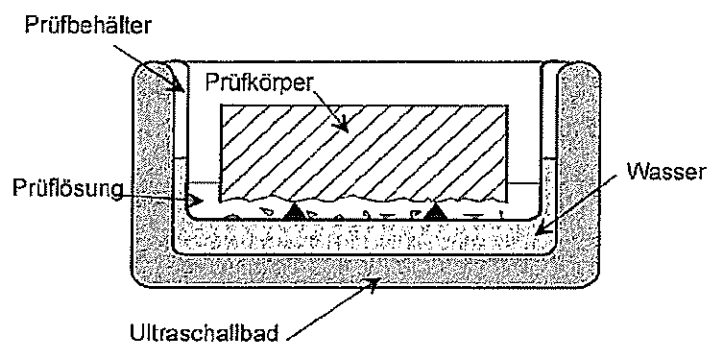
Abbildung 6: Ultraschallbad
