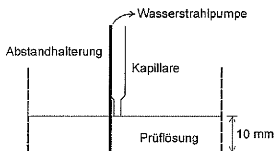
Abbildung 5: Absaugeinrichtung
