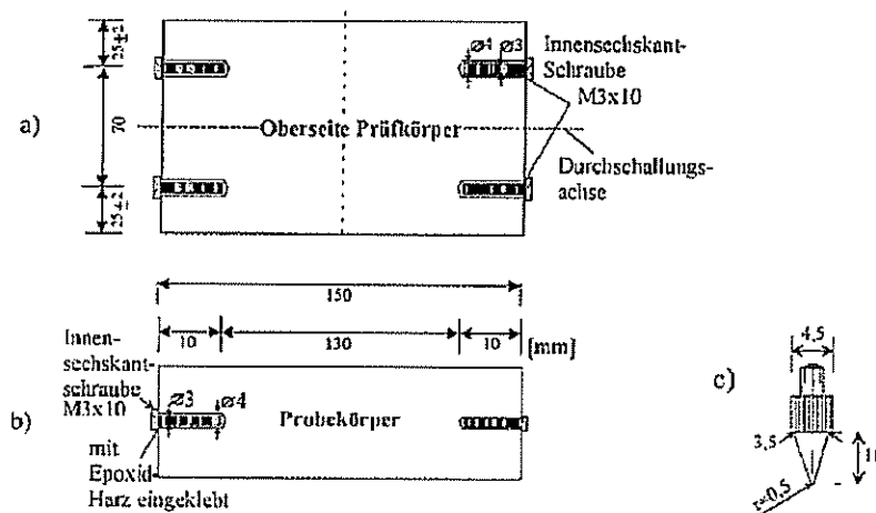
Abbildung 10: Prüfeinrichtung zur Messung der Längenänderung
