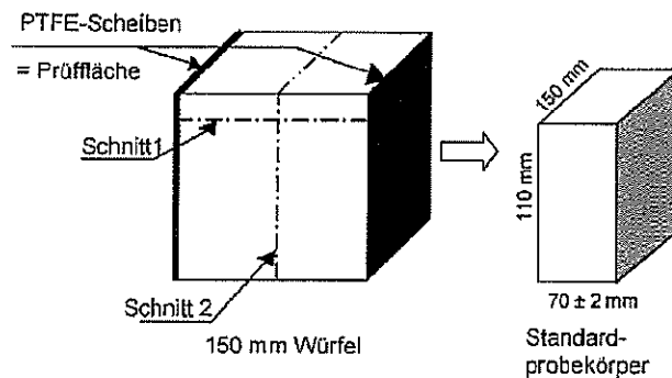
Abbildung 7: Zusägen der Probekörper bei seitlicher PTFE-Scheiben Anordnung
