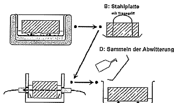
Abbildung 8: Messabfolge mit Referenzmethode
