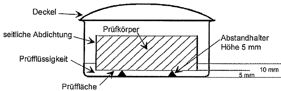
Abbildung 1: Kapillares Saugen
