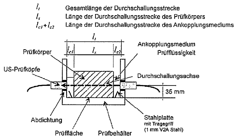
Abbildung 9: Messaufbau zur Bestimmung der Ultraschalllaufzeit
