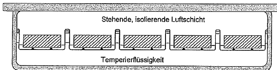
Abbildung 3: Temperaturkontrollierte Truhe
