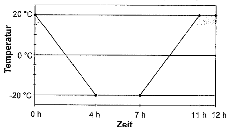
Abbildung 4: Kontrolltemperatur-Zyklus
