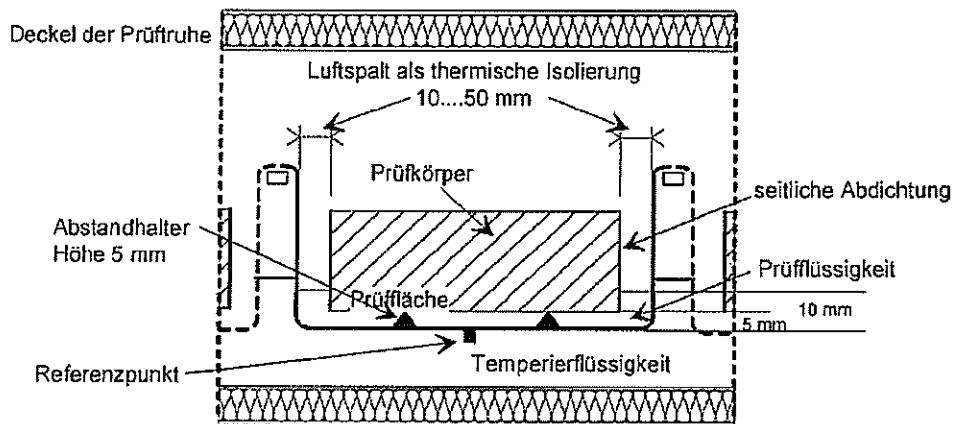
Abbildung 2 : Prüfbehälter mit Probekörper im Flüssigkeitstemperierbad
